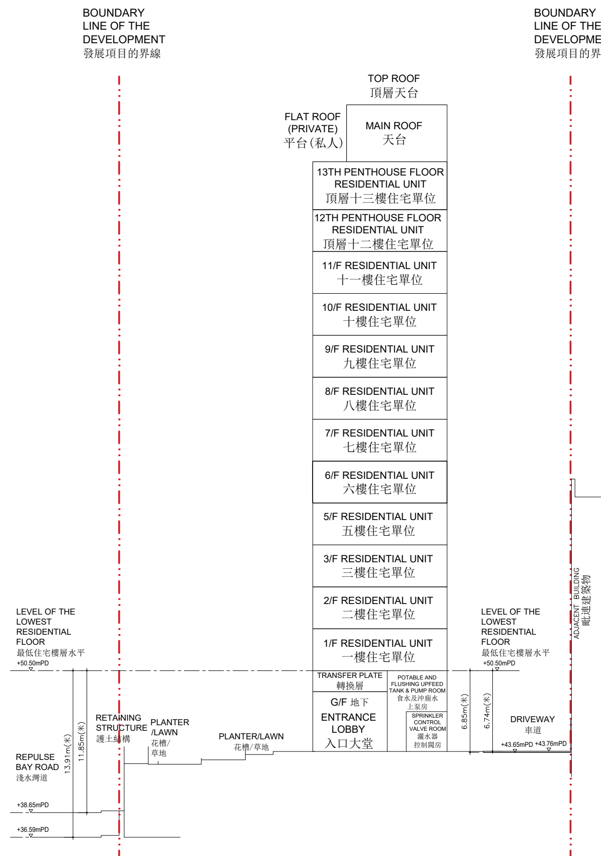
CROSS-SECTION PLAN B-B 橫截面圖 B-B
